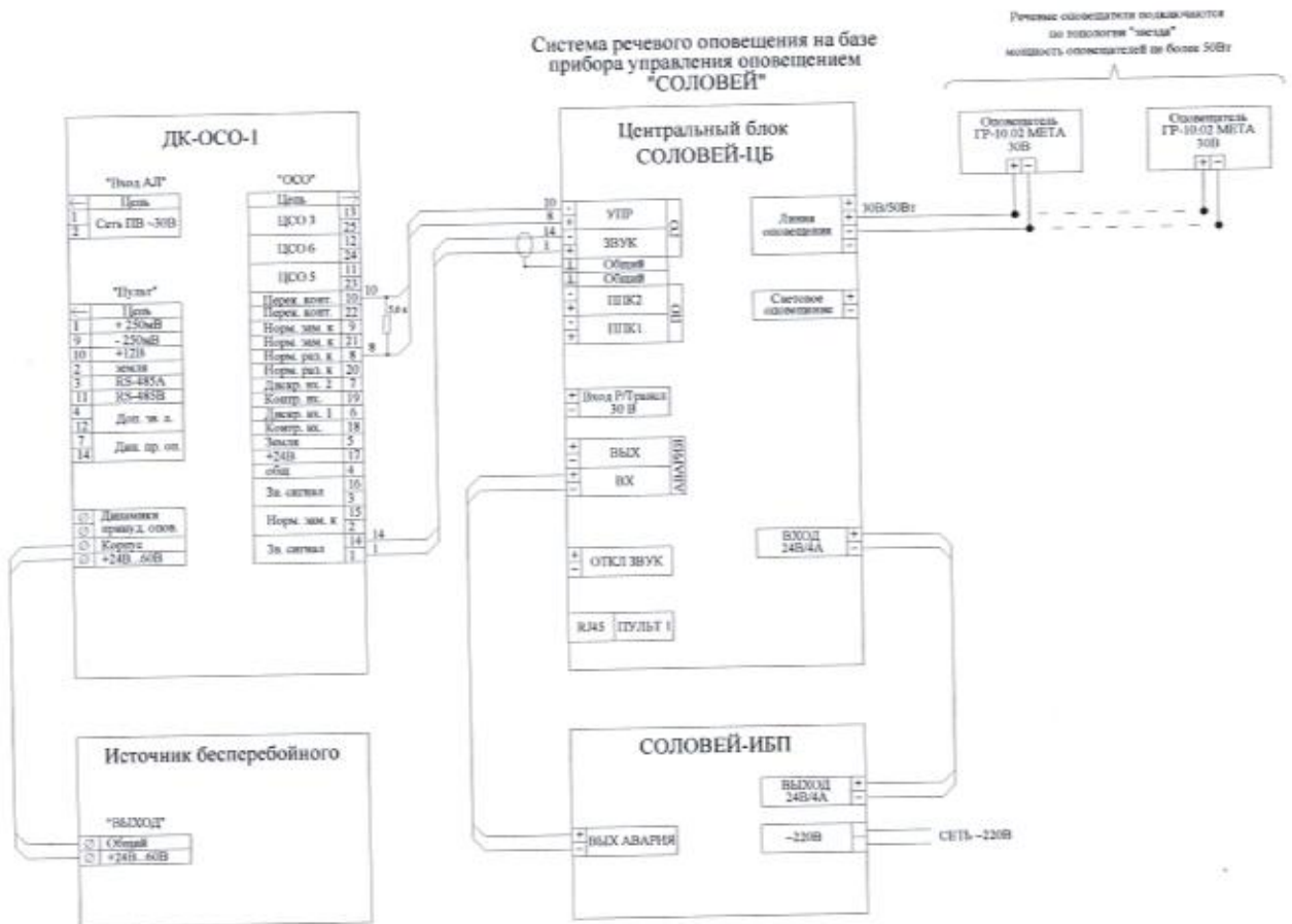
Рис. 2. Схема подключения к РАСЦО по сети проводного вещания.
